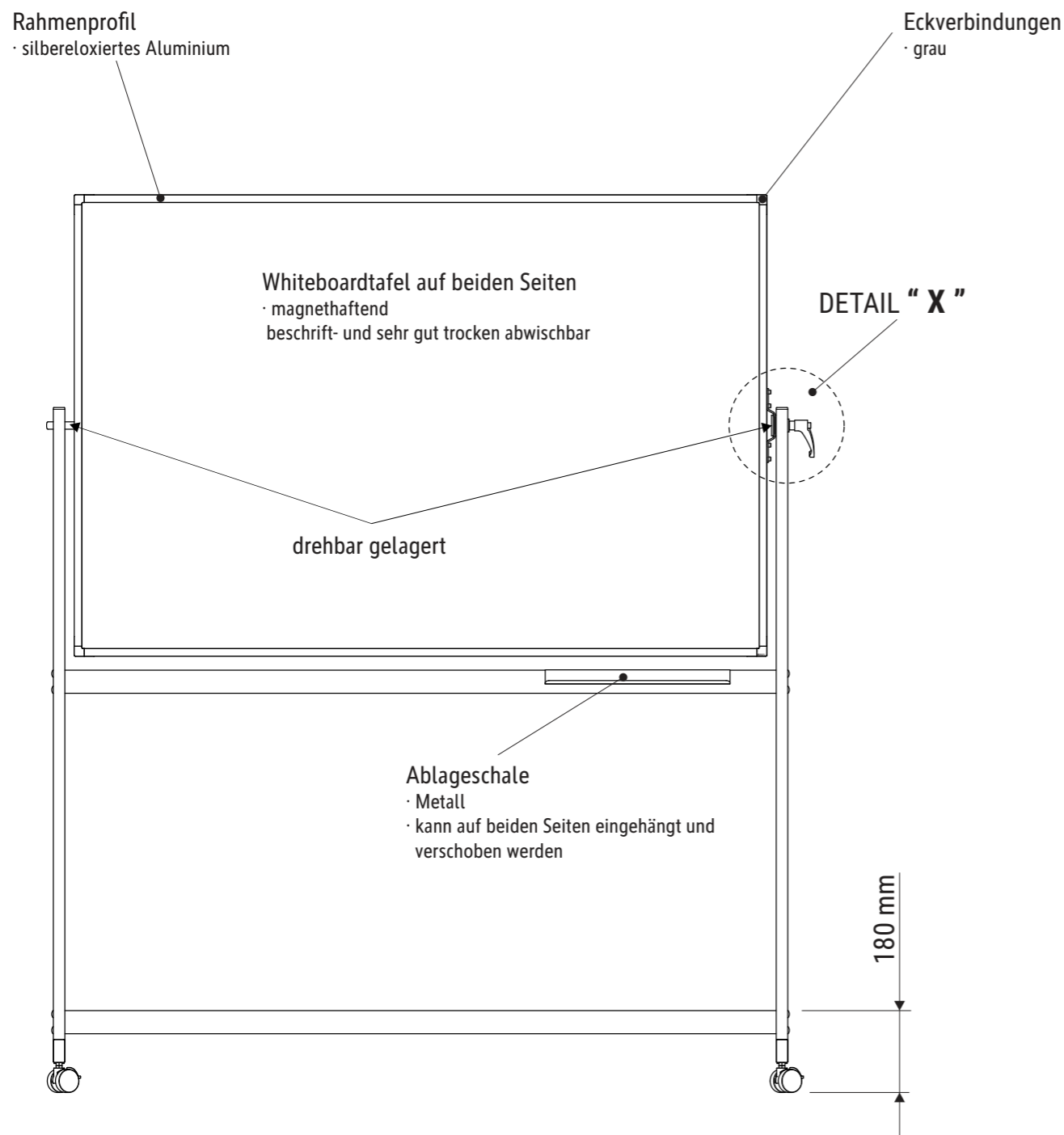
Detail „X“
