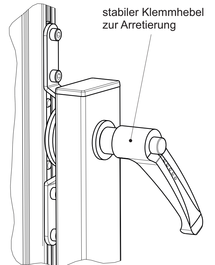
Detail „X“
