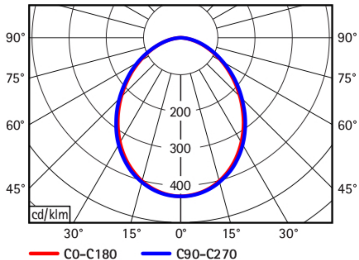
Lichtverteilungskurve
