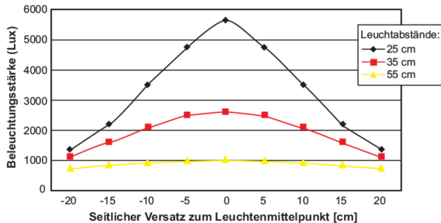
Beleuchtungsstärke in Abhängigkeit vom Abstand
